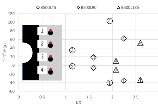
図-6 ひずみー l/D (150kN 時)
