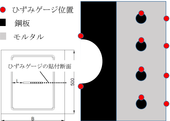
図-2 ひずみゲージの貼付位置
