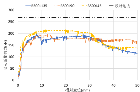
(a) 有孔鋼板と補強筋までの距離による影響
