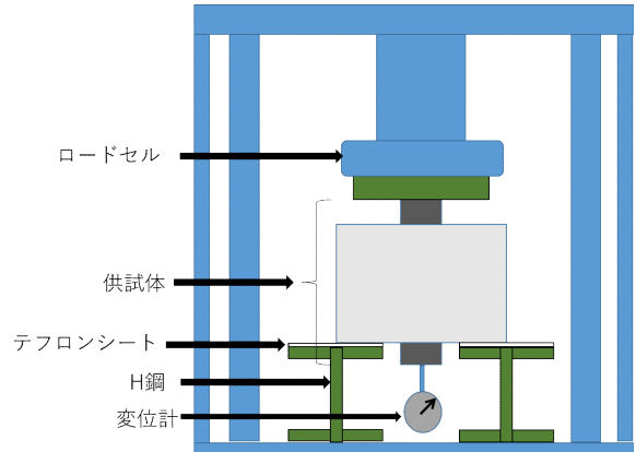
図-3 試験方法
