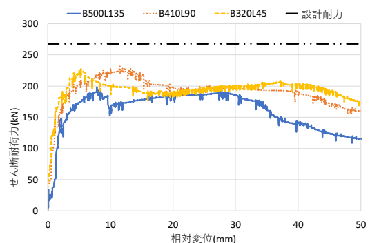
(b) モルタルブロックの寸法による影響
