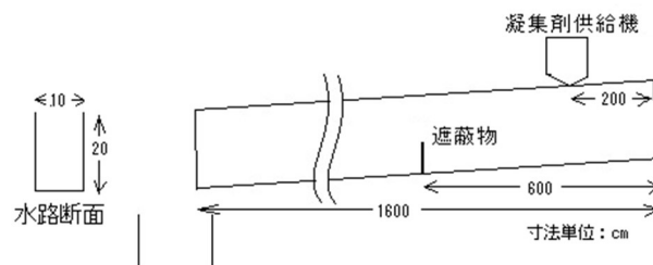
図-2 実験水路図
