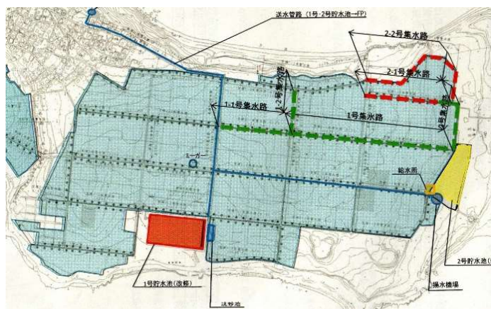
図-1 津堅島農村基盤整備事業水利施設整備図
