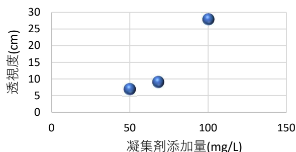
図-3 凝集剤添加量と透視度の関係
