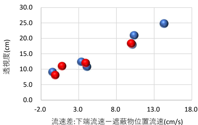
図-5 遮蔽物による流速差と透視度の関係
