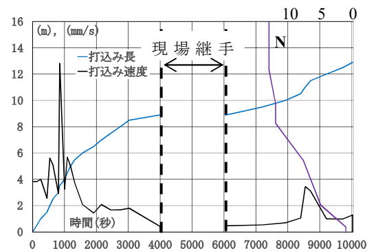
図-2 打ち込み長さ，速度の時刻履歴
