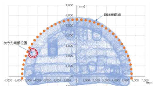
図－3 カッタヘッド軌跡表示例
