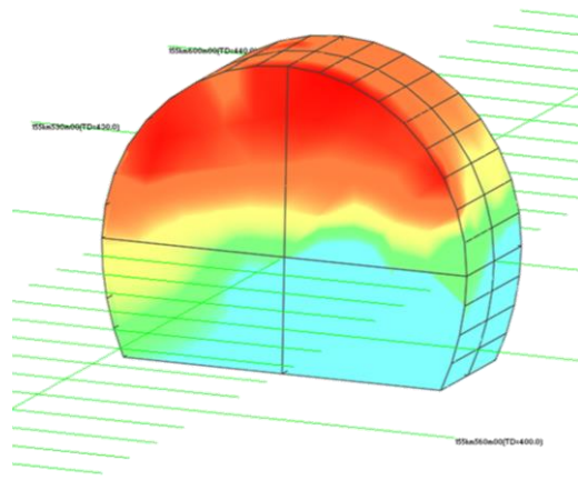
図－4 地山強度による評価例
