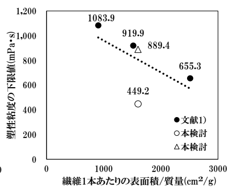
図-4 繊維の表面積質量比と塑性粘度の下限値
