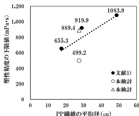
図-3 繊維の平均径と塑性粘度の下限値
