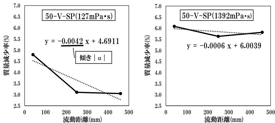
図-1 流動距離と質量減少率（平均径 48.7\mu\text{m} ）
