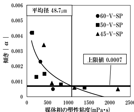
図-2 媒体相の塑性粘度と傾き |\alpha|
