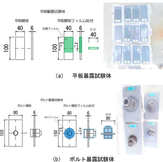
図-2 暴露試験体
