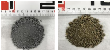
写真-1 石炭灰混合破碎材の外観 写真-2 一般盛土材の外観
