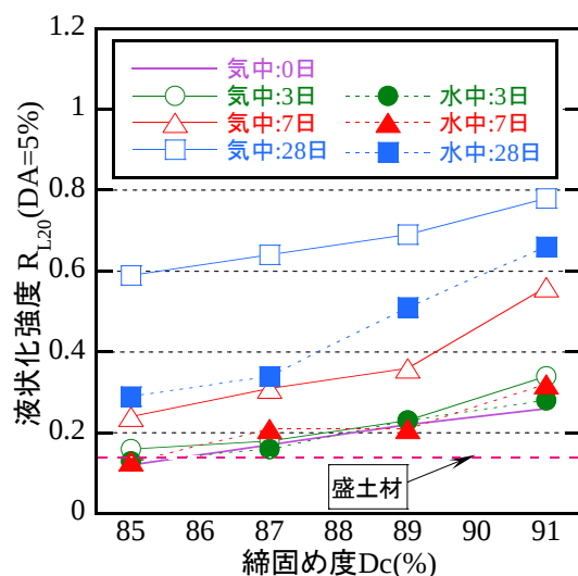
図-6 予測した液状化強度
