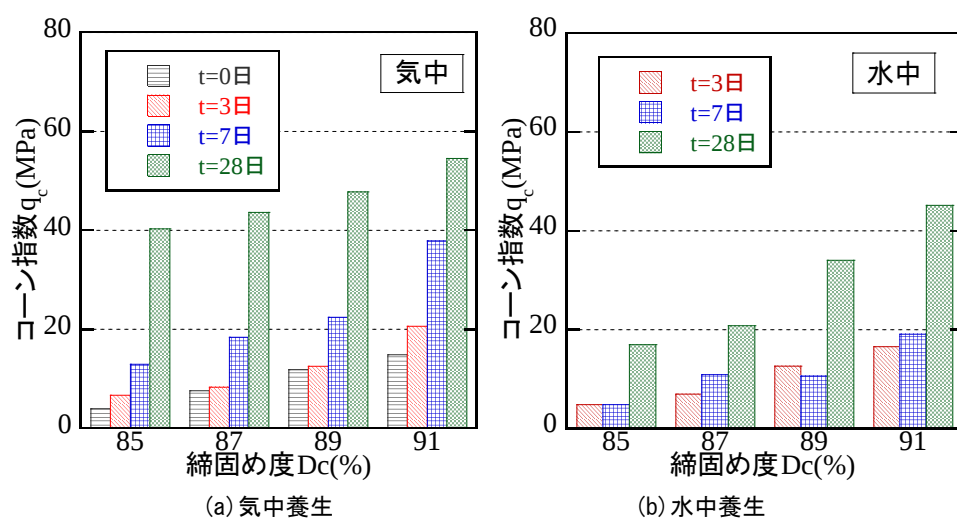
図-4 コーン指数に及ぼす締固め度の影響
