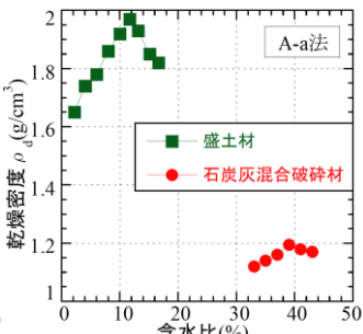
図-2 締固め度曲線
