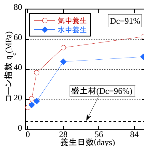
図-3 コーン指数に及ぼす自硬性の影響
