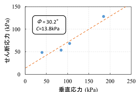
図 8 ピーク時の応力値のプロット
