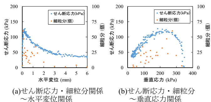
図 7 初期垂直応力 400kPa の試験結果
