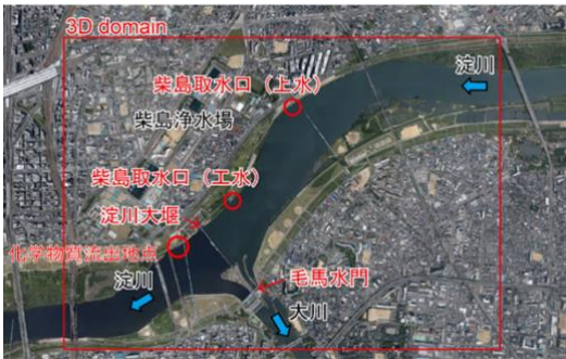
図 1 三次元解析領域および仮想の化学物質流出地点
