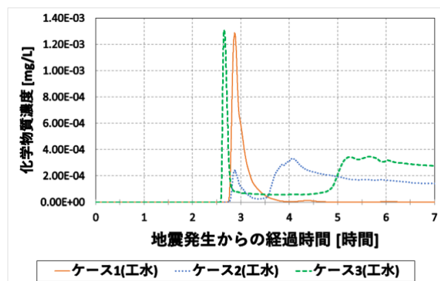
図5 化学物質濃度の時間変化
