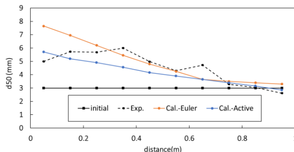
図-4 表層のd50の縦断分布
