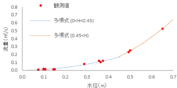
図 3.2-H-Q 曲線式
