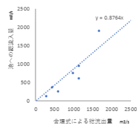
図 4.2.3-合理式による総流出量と池への総流入量の関係
