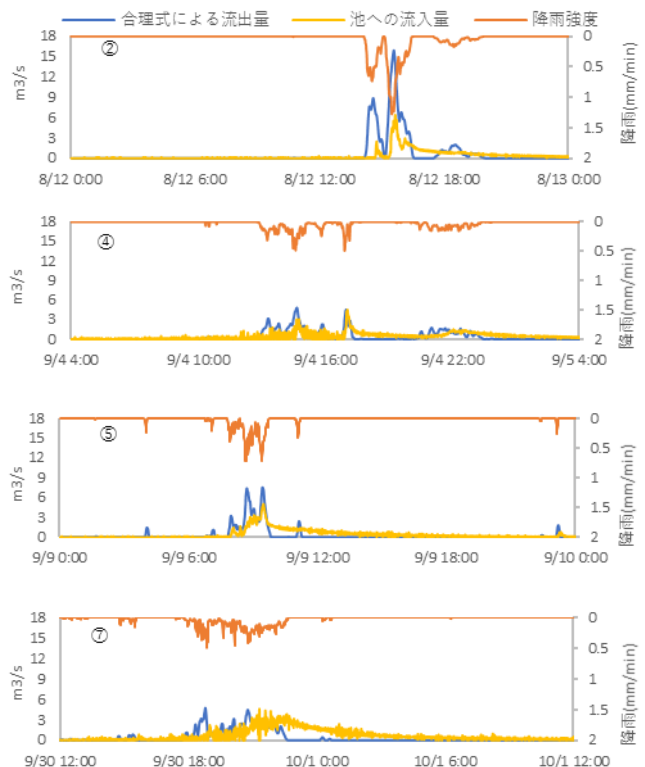
図 4.2.2-ハイドログラフ
