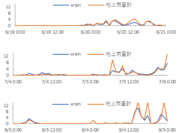
図 4.1-地上雨量と XRAIN データの比較
