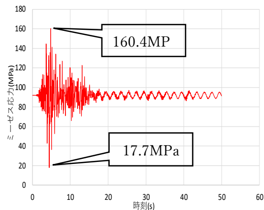
図-5 補強材接続部時刻歴応答ミーゼス応力
