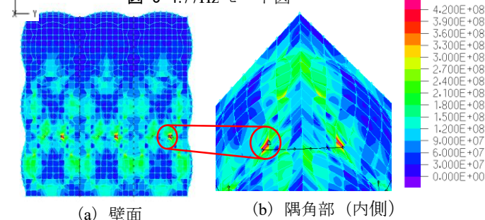
図-4 ミーゼス応力 (分布図)
