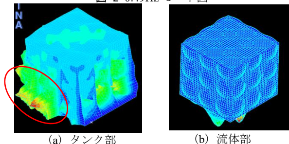
図-3 4.77Hz モード図
