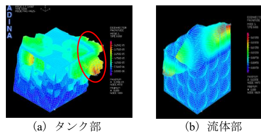
図-2 0.49Hz モード図
