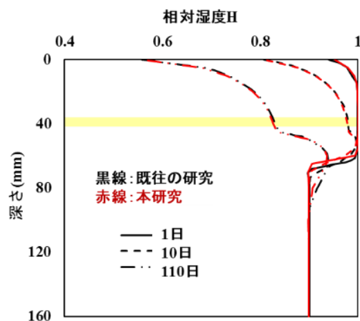
図-2 相対湿度分布
