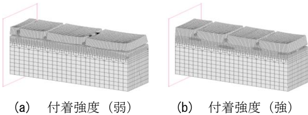
図-3 ひび割れ分布
