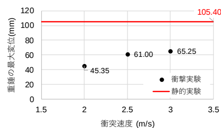
図-6 最大変位の比較 (MDPE 管)
