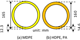
図-2 管の断面寸法
