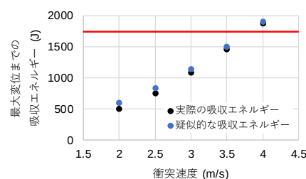
図-8 吸収 E の比較 (HDPE 管)
