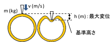
図-5 吸収エネルギーの算出 (衝撃試験)
