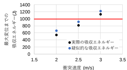
図-7 吸収 E の比較 (MDPE 管)
