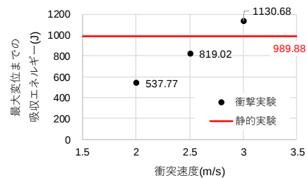
図-4 吸収エネルギーの比較 (MDPE 管)
