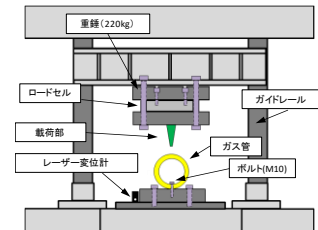
図-1 落錘式衝撃実験装置
