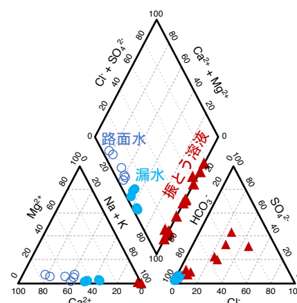
図 7 振とう溶液と漏水と路面水のトリリニアダイアグラム。
