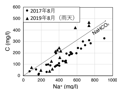
図 6 振とう溶液の pH と無機 C 濃度の関係
