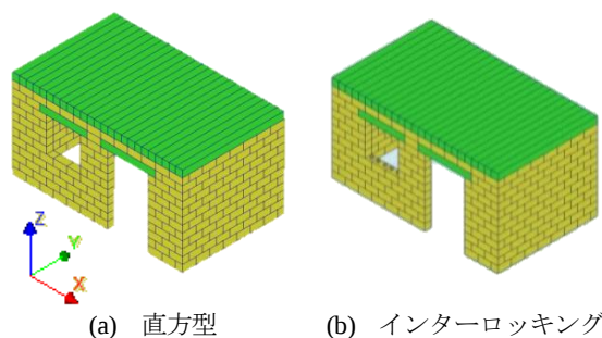
図2 建物のモデル
