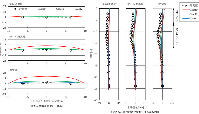
図-5 弾性係数の影響
