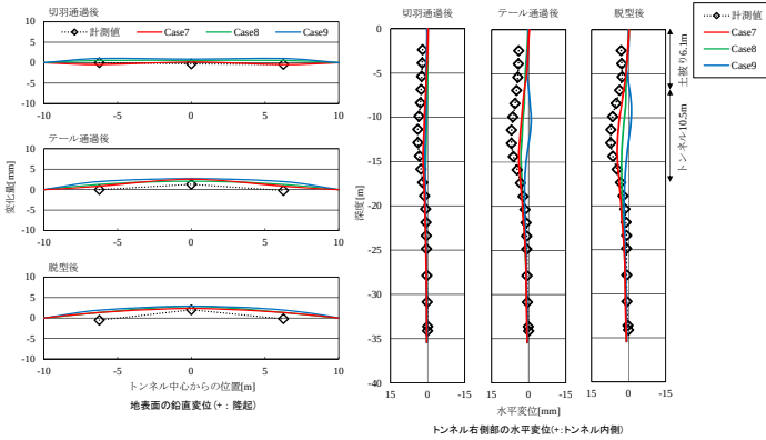
図-4 静止土圧係数の影響
