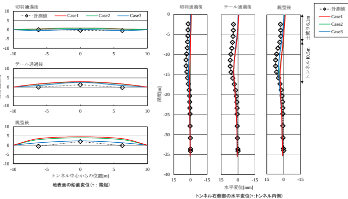
図-3 初期変位の影響
