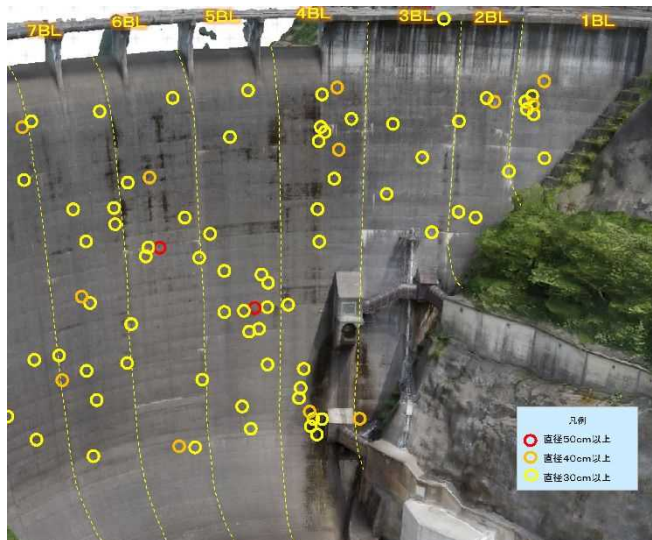
図-7 ディープリンングにより検出されたポップアウト位置（下流面：φ30cm 以上を抽出）
