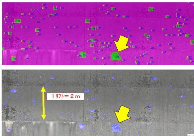
図-3 検出されたポップアウトのうち最大のものの（ \phi 57.4\text{cm} 、堤体 5 ブロック下流面）
