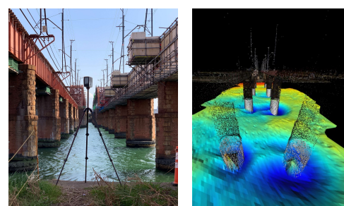
(a) スキャニングソナー測量 (b) 点群データ
