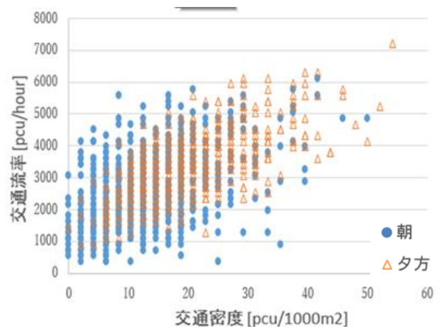
図-2 交通流率と交通密度の関係
