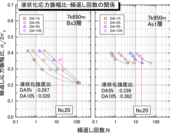
図-4 液状化強度特性曲線
