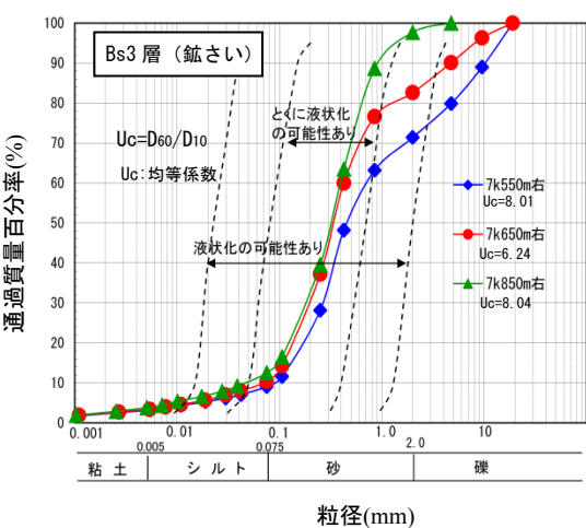
図-3 粒径加積曲線 (Bs3 層)
