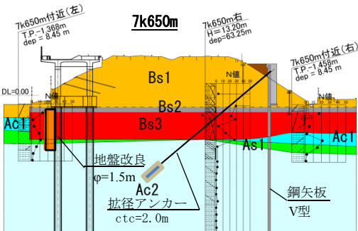
図-5 耐震補強断面図
