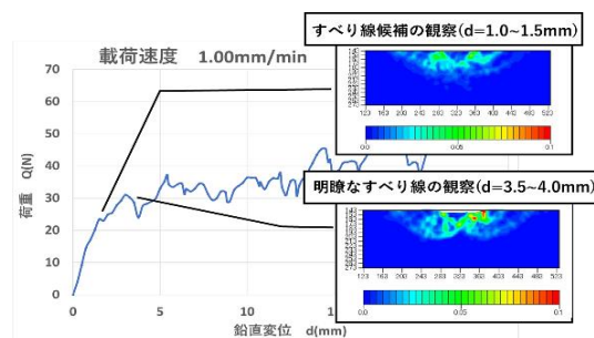
図 3. すべり線の観察
