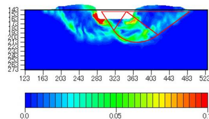
図 5. 最大せん断ひずみの分布図と支持力理論曲線
