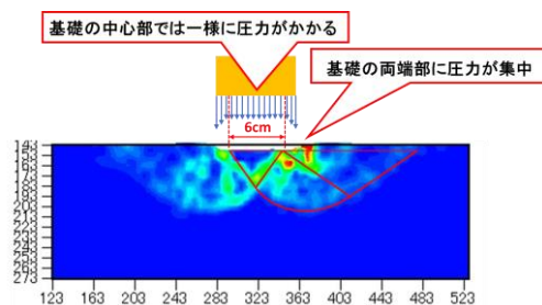
図 6. すべり線形成範囲の考察
