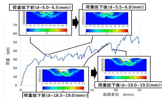
図 4. 荷重の増加・減少
