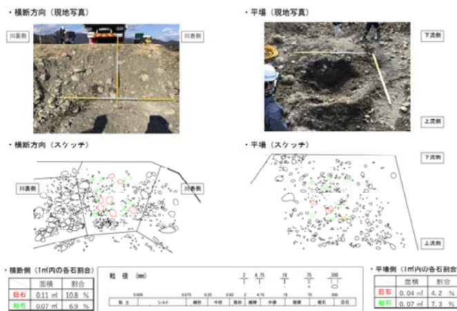
図4 2019 年開削調査結果/盛土上部
