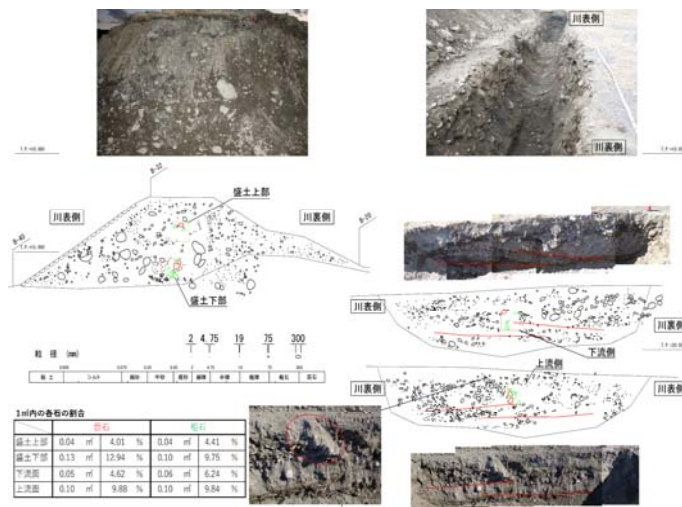
図1 2017年開削調査結果/左:盛土部, 右:基礎地盤
