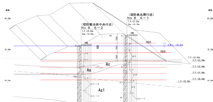
図2 開削調査断面, 既往ボーリング調査と設定モデル
