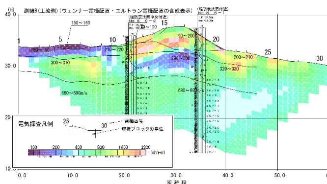
図3 物理探査結果図
