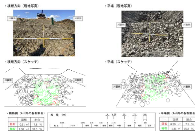
図5 2019 年開削調査結果/盛土下部
