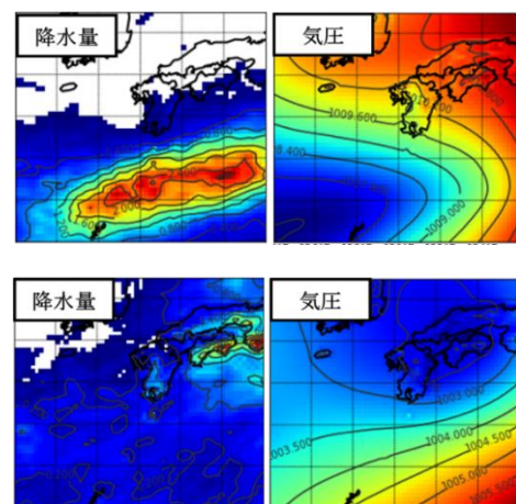
図-5 「将来増加型」(上)と「将来減少型」(下)の降水量(左)と気圧(右)の空間分布図
