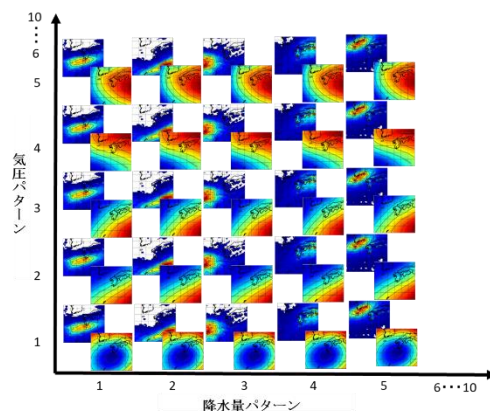
図-3 降水量（横軸）と気圧（縦軸）の2次元マップ
