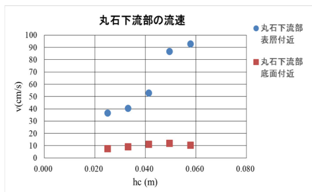
図1 丸石下流部における表層, 底面付近の流速変化
