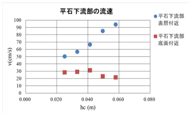
図2 平石下流部における表層, 底面付近の流速変化
