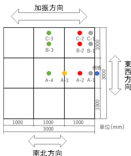
図-1 水圧センサー設置位置（上面図）
