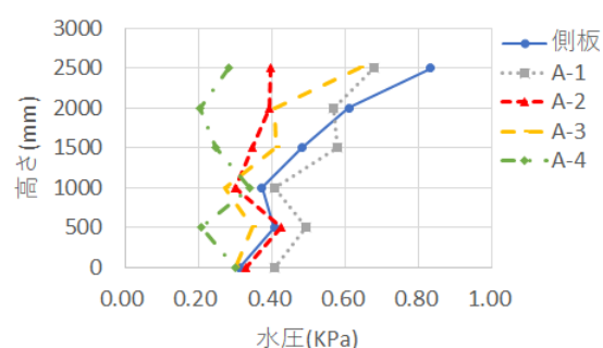
(a) スロッシング1次モードA面
