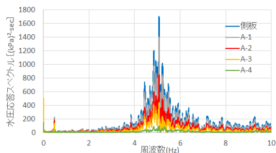
図-3 水圧応答スペクトルー振動数関係 (東北地方太平洋沖地震(変位20%相当))
