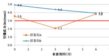
図-9 引張試験結果 (下向き設置)
