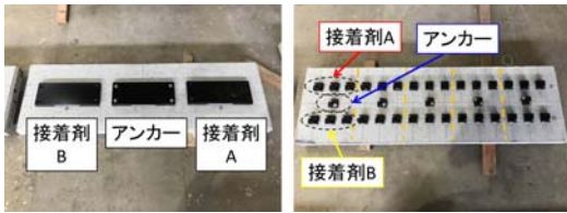
図-4 作成した供試体 (左：加振試験用 右：引張試験用)
