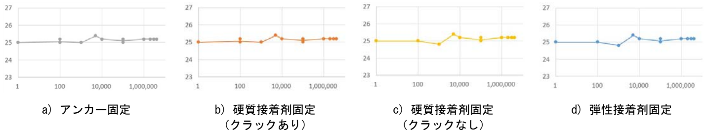
図-7 初回～400 万回のピーク周波数の推移(横軸：载荷回数，縦軸：周波数)
