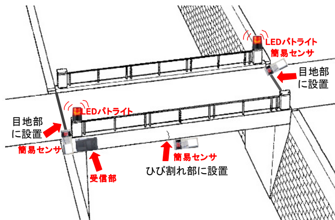
図-3 簡易センサの適用例
