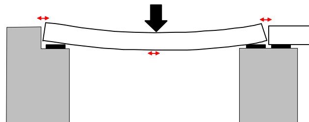
図-2 桁たわみと桁端部挙動の関係
