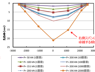
図-6 主桁のたわみの推移
