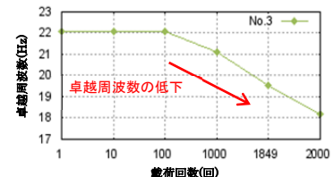
図-8 卓越振動数の推移 2)
