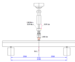
図-2 疲労・静的載荷試験の装置図と外観
