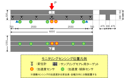
図-4 センサの配置図
