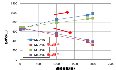
図-7 载荷回数と主筋ひずみの関係
