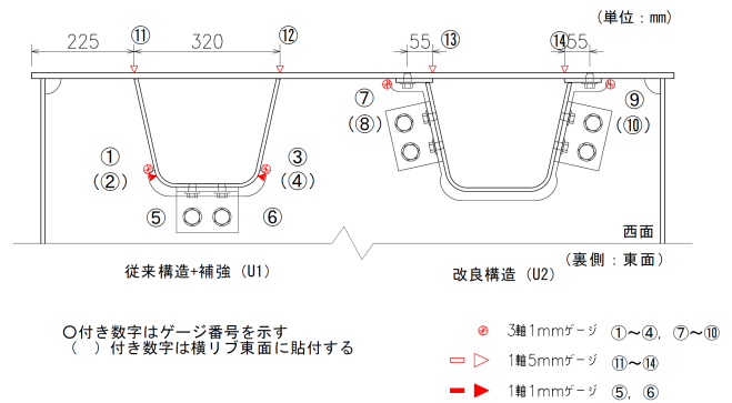
図-2 スクラップ部詳細とひずみゲージ貼付け位置
