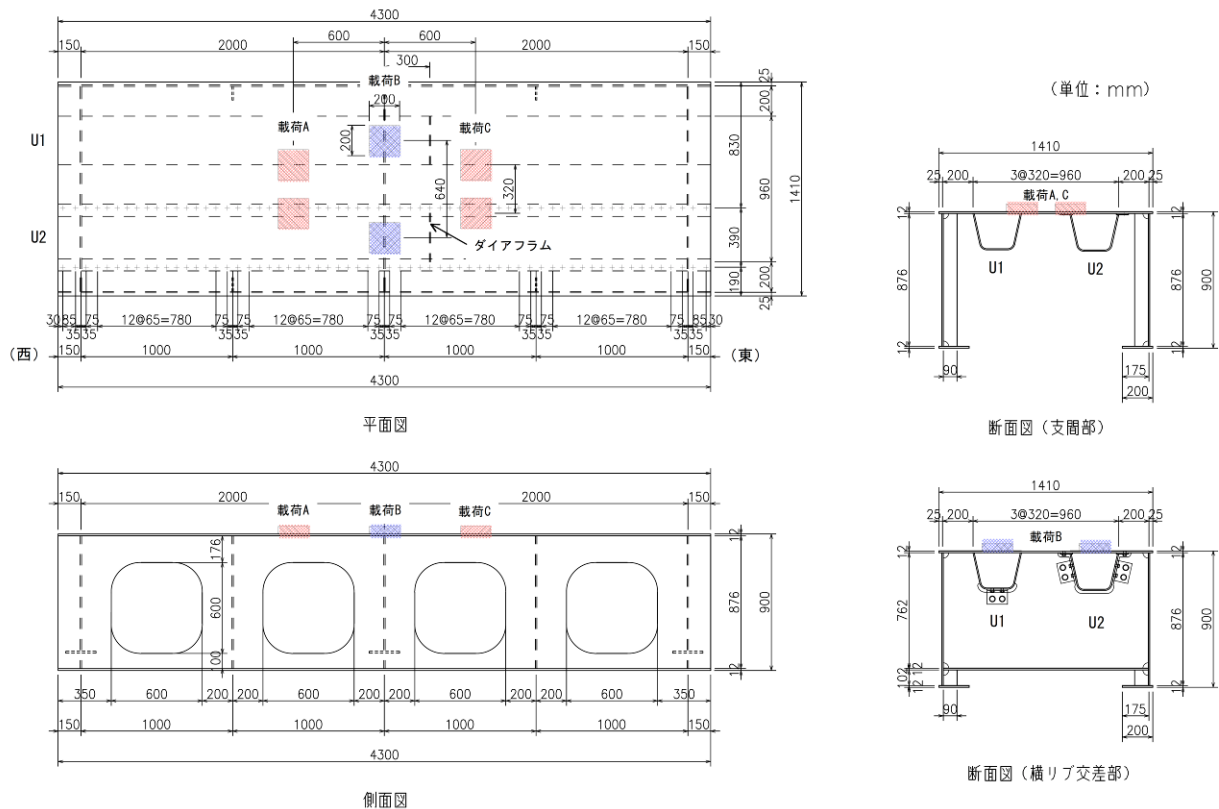
図-1 試験体の寸法と形状、载荷位置
