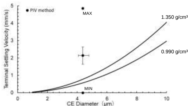
図-4 ストークス則(実線)と PIV 法(点)による沈降速度の比較
