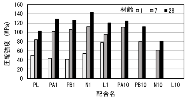
図-1 セメントペースト圧縮強度
