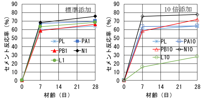
図-2 セメント反応率
