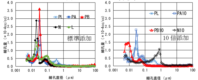
図-3 材齢 28 日の細孔径分布
