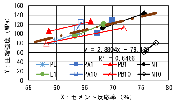
図-4 セメント反応率と圧縮強度
