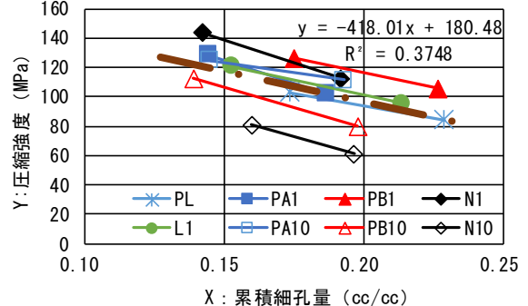
図-5 累積細孔量と圧縮強度
