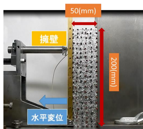
図-1. 変形前の擁壁とアルミ棒積層体
