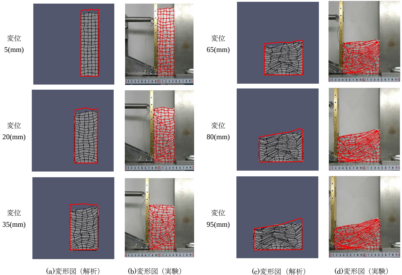
図-3. 実験と数値解析の変形比較図
