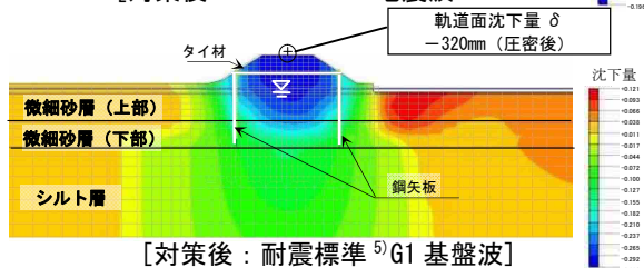
図-4 軌道面沈下量の比較 (No. 1 安食・小林間)
