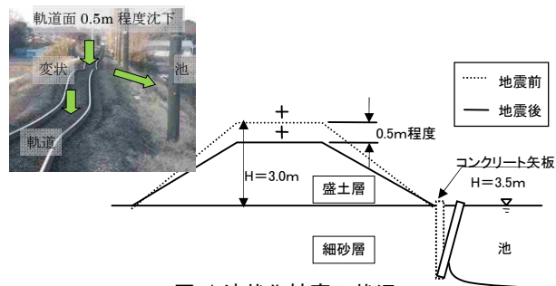
図-1 液状化被害の状況
