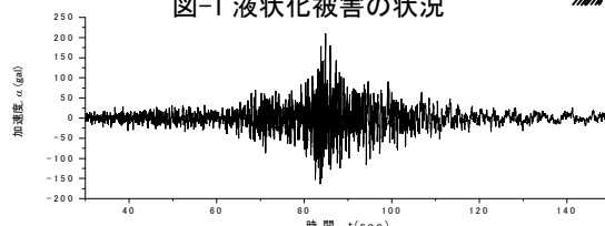
図-2 入力地震動(作成した基盤波形)
