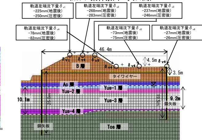
図-9 解析モデルと対策後の最大沈下量 (No.5 金町・松戸間)
