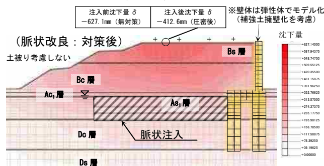
図-6 解析モデルと対策後の最大沈下量(No.2 小岩・市川間)
