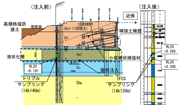
図-5 サンプリング位置図・柱状図(No.2 小岩・市川間)
