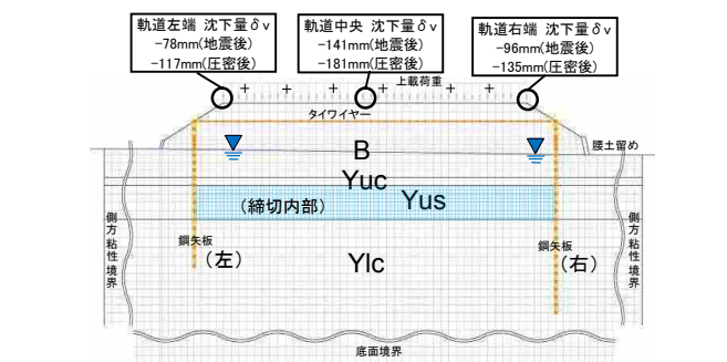
図-7 解析モデルと対策後の最大沈下量(No.3 赤羽・川口間)
