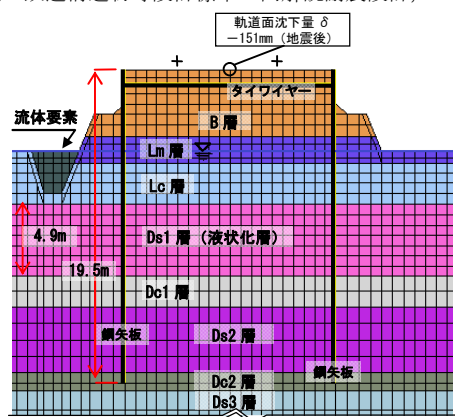
※洪積層のため、地震後の圧密沈下は考慮していない。 図-10 解析モデルと対策後の最大沈下量 (No.6 大宮操車場)
