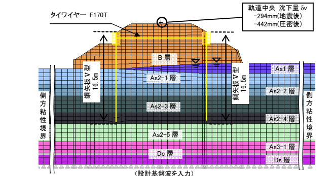
図-8 解析モデルと対策後の最大沈下量 (No.4 東神奈川・大口間)
