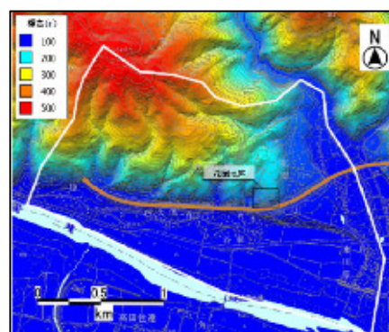
図.3 検討範囲平面図
