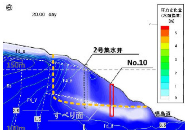
図.8 豪雨時解析結果図
