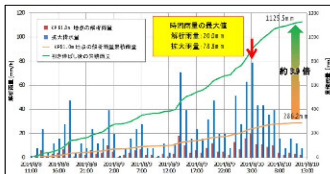
図.7 豪雨時 雨量波形
