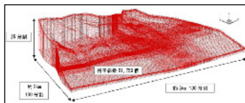
図.4 計算格子鳥瞰図
