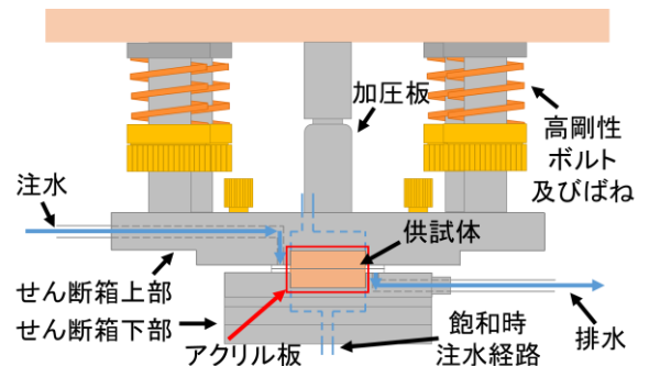
図1 一面せん断試験機
