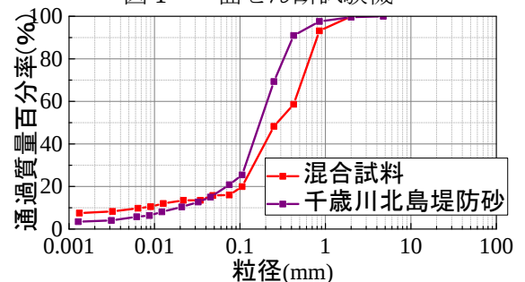
図2 試験試料の粒度分布
