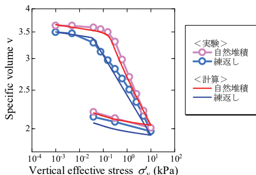
図 2 標準圧密試験結果と計算結果
