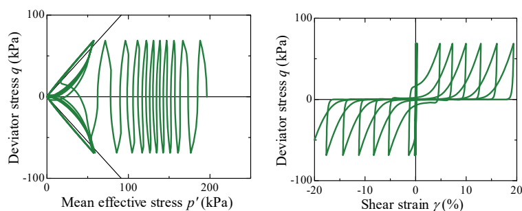
図 1 複合負荷弾塑性構成式による砂の液状化試験のシミュレーション例
