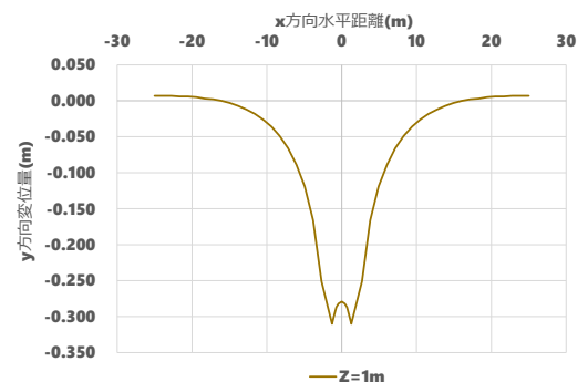
(a) 引抜孔が空洞の場合
