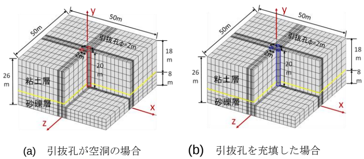
図-1 解析断面
