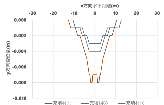
(c) 充填材①、②、③を充填した場合
