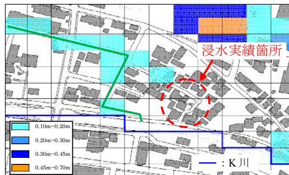
図4 内水氾濫解析結果(CASE2)
