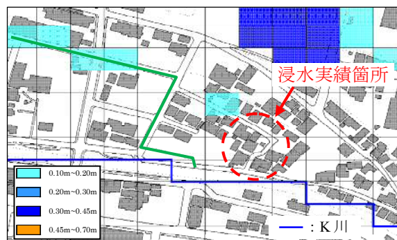
図6 内外水氾濫解析結果(CASE4)
