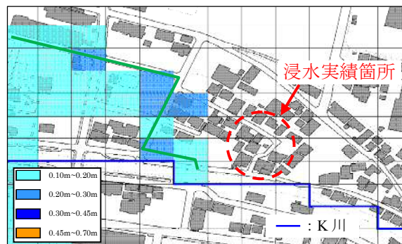
図3 外水氾濫解析結果(CASE1)
