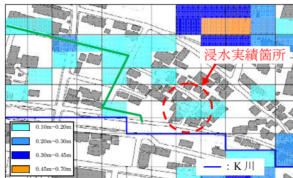
図5 内外水氾濫解析結果(CASE3)
