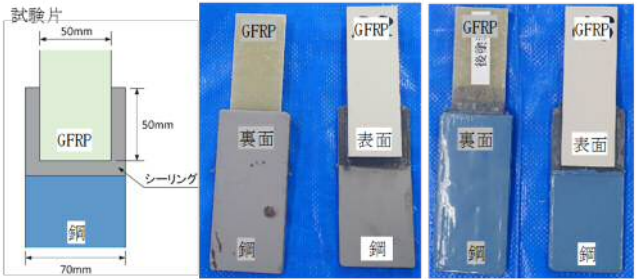
(a)試験片図
