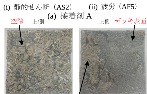
写真-1 破壊面の状態の例
