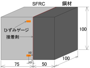
図-1 試験体の寸法形状
