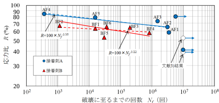
図-3 セン断疲労試験結果 (S-N 関係)
