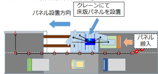
図-1 既存RC床版更新の施工ステップ
