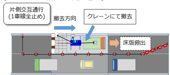
【ステップ1：既存 RC 床版の撤去】
