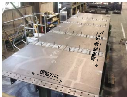
(a) 床版パネルの地組立
