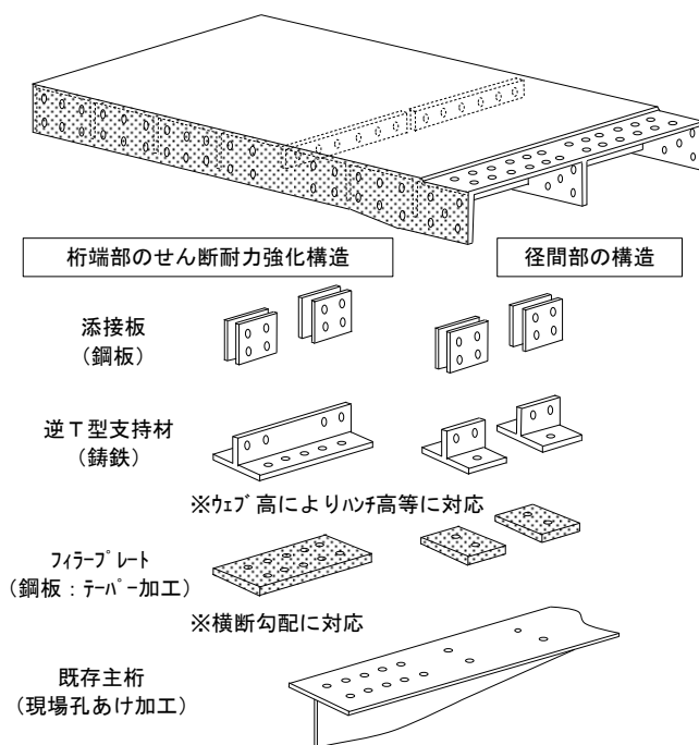
図-2 主桁との連結構造
