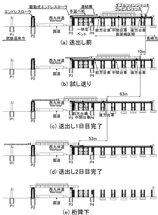
図-3 中央径間の架設ステップ図
