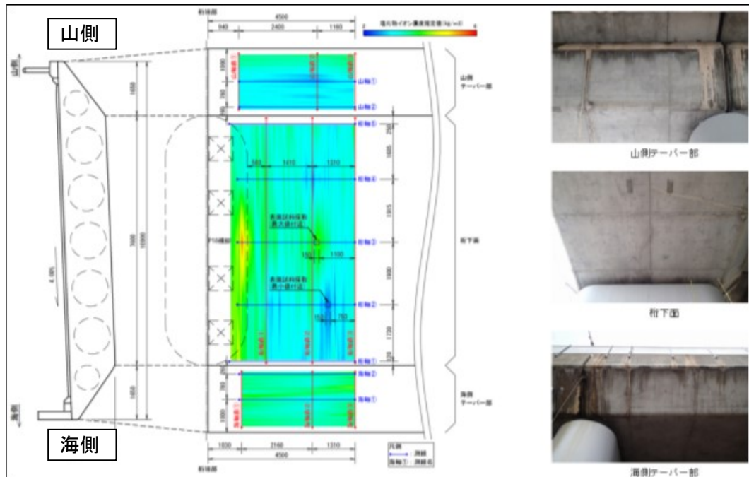
図 2 近赤外線法によるコンクリート表面塩分分布測定結果
