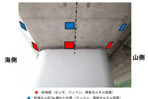
写真 2 センサ、ワッペン、薄板小型モルタルの設置位置
