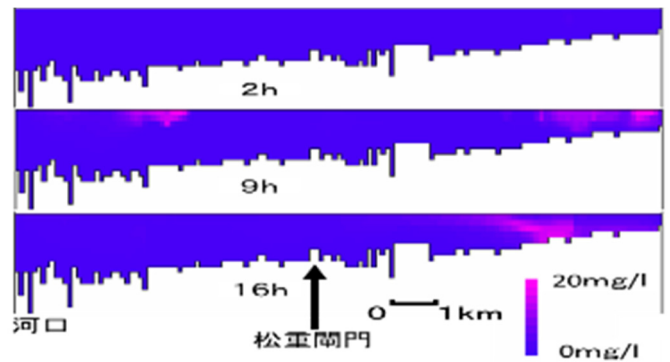
図-4 堀川における SS の分布
