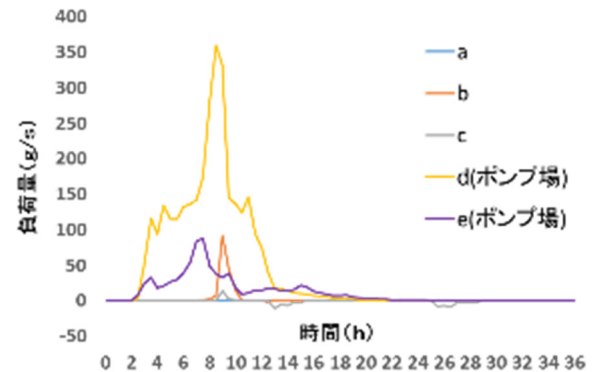
図-5 堀川へ流入する負荷量の時間変化
