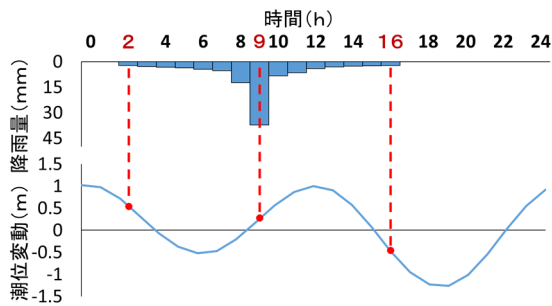
図-2 計算条件および潮汐
