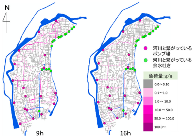
図-3 下水道内の汚濁負荷量
