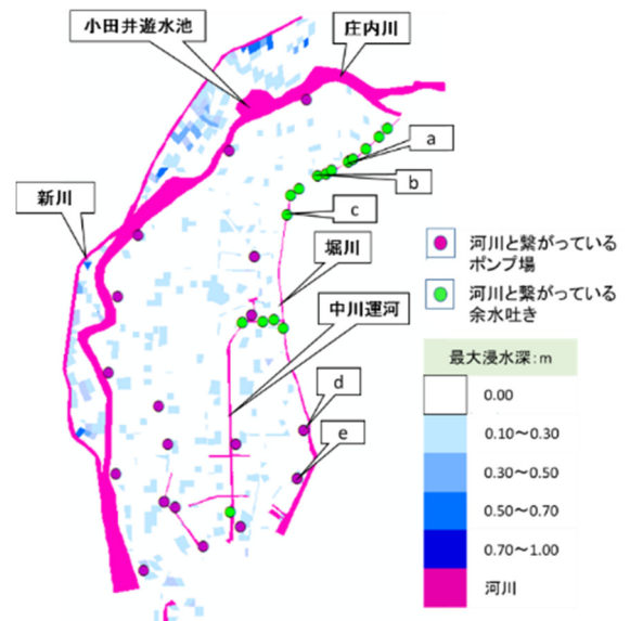
図-1 計算領域と最大浸水深の分布
