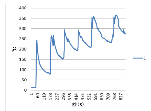
図 4. CASE.0 裏面温度
