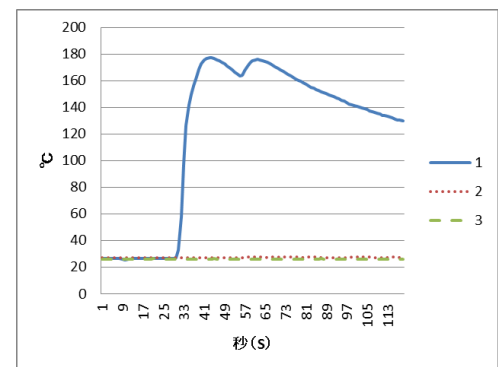
図 3. CASE.1 裏面温度
