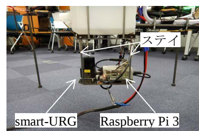
写真 3. 測域センサ
