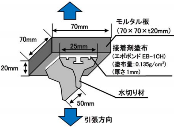
図-1 接着性試験の概要
