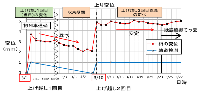
図-5 桁と軌道の計測結果
