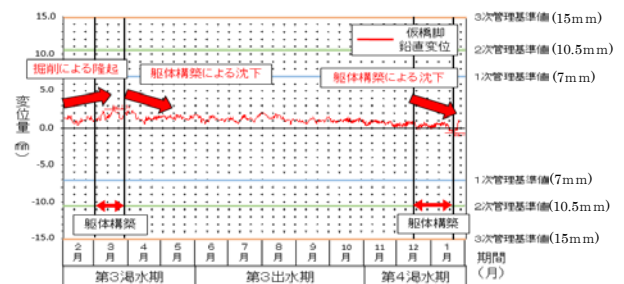
図-6 新設橋脚構築時の変位
