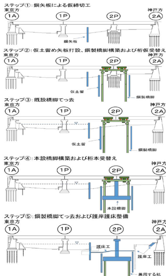
図-2 施工ステップ
