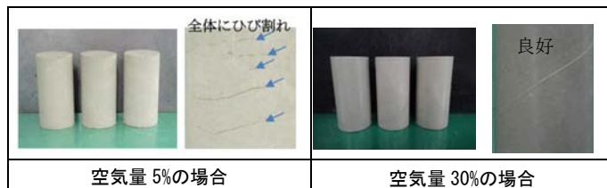
写真-2 試験ケース 3-1 での供試体表面
