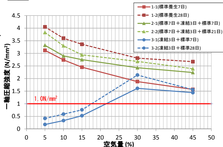
図-1 各養生条件での空気量と一軸圧縮強度との関係
